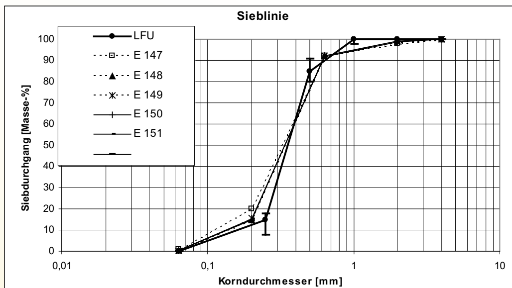
Überprüfung der Kornverteilung eines Filtersubstrates
